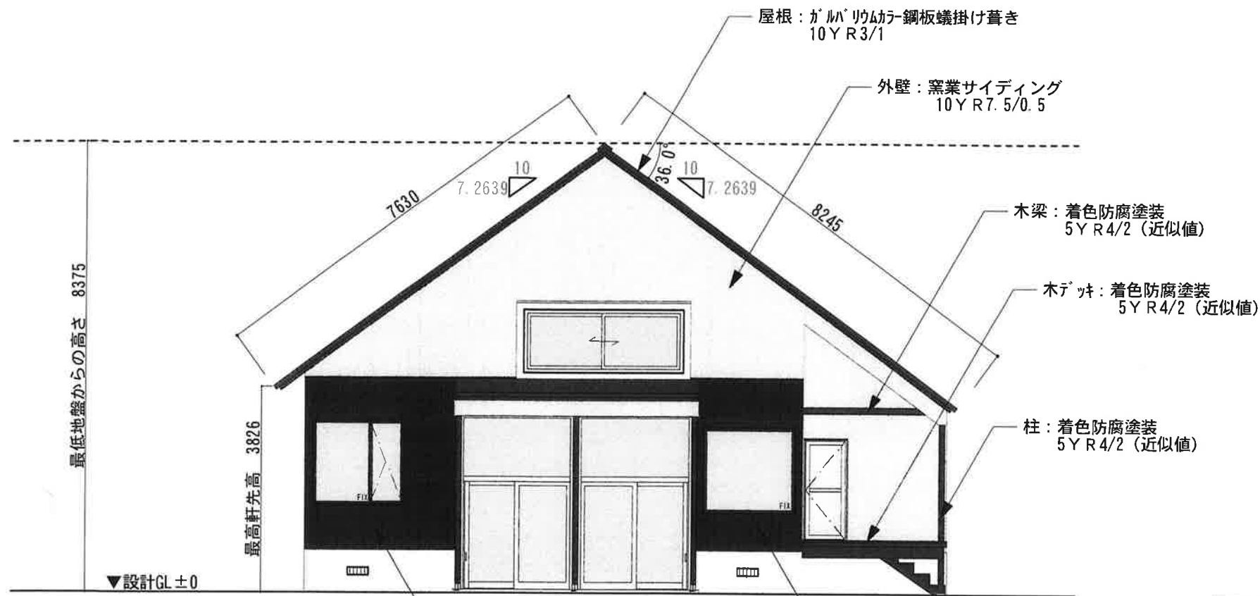
南側立面図
