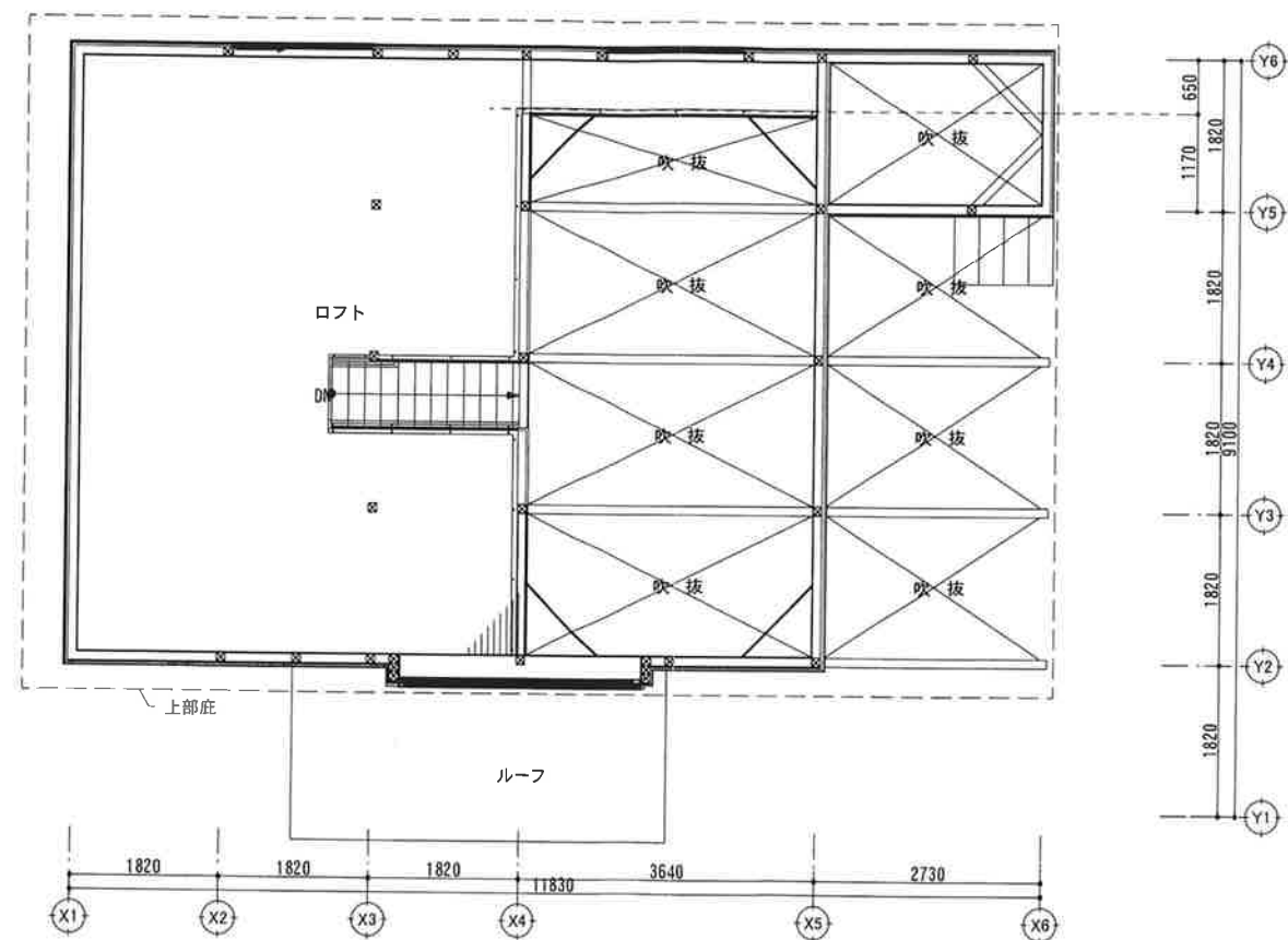
2階 平面図
