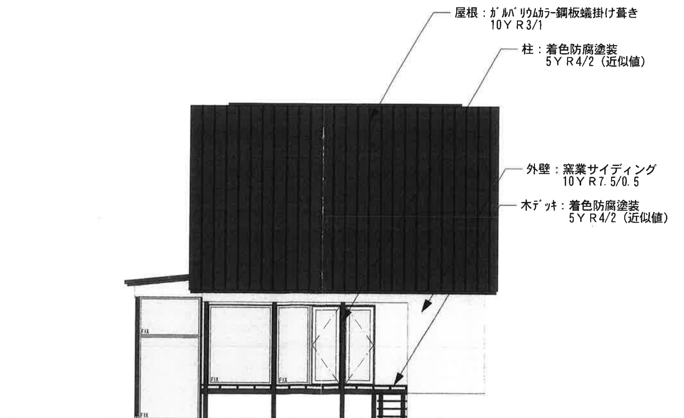
東側立面図
