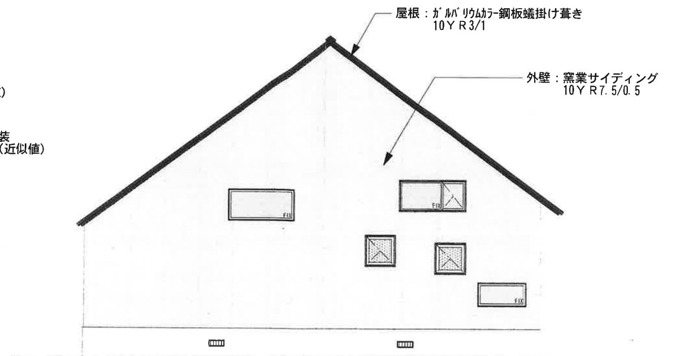
北側立面図
