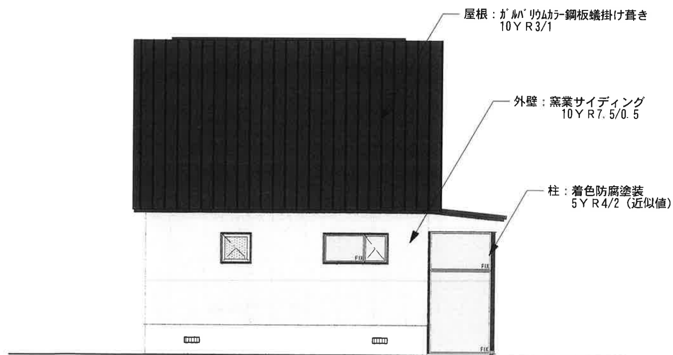
西側立面図
